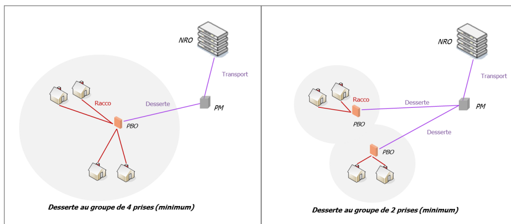
Figure 17 : Schéma descriptif d'une architecture au groupe de deux prises et au groupe de quatre prises
