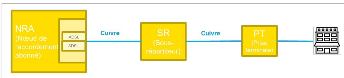
Figure 3 : Architecture du réseau cuivre
