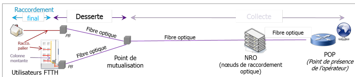
Figure 2 : Architecture du réseau FttH
