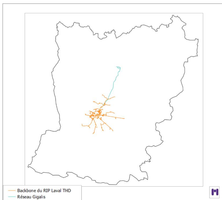
Figure 12 : Réseau Gigalis et Backbone du RIP Laval THD
