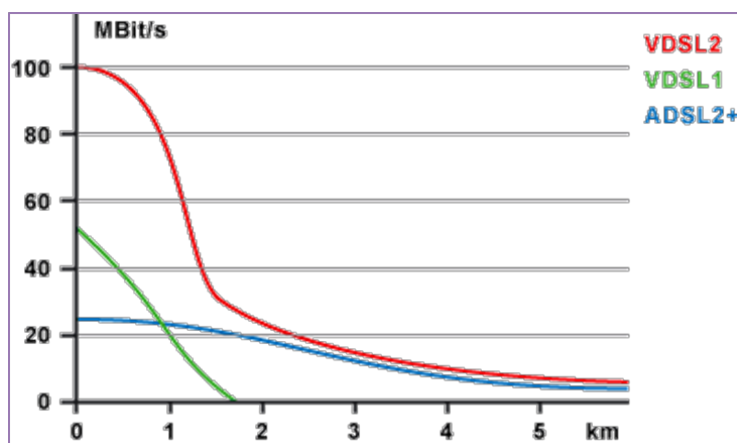
Figure 4 : Impact de distance abonné-PT au NRA sur la qualité du débit
