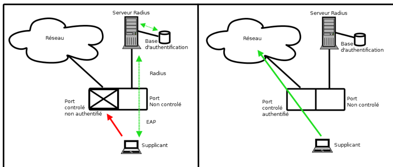
Figure 1 : Authentification 802.1X avec Radius
