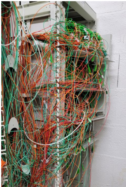
Illustration de la non-conformité des raccordements à Saint-Julien-en-Genevois. Chaque câble correspond à un client.
